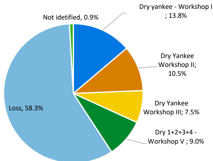
Hình 1. Biểu đồ phân bố lượng nhiệt sử dụng trong Nhà máy
